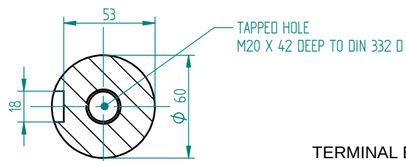
Przekrój A-A 1:2
